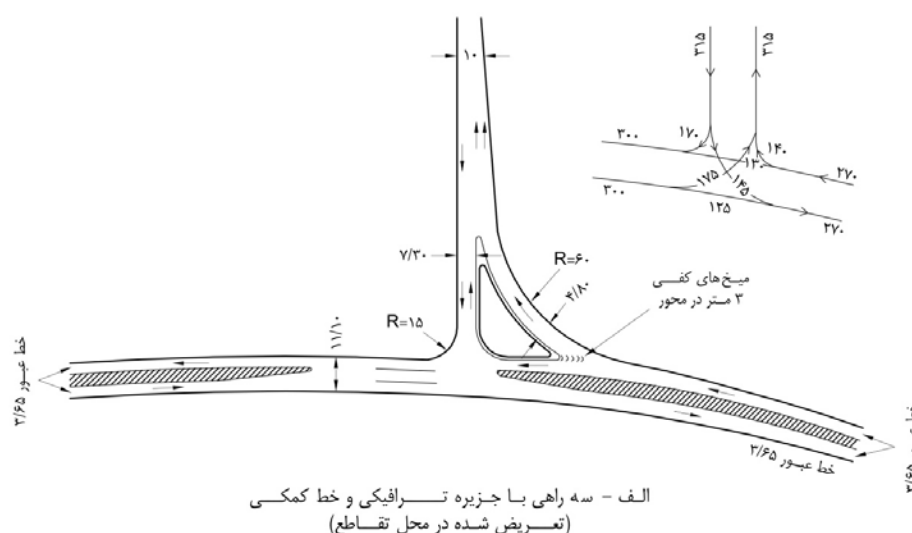
شکل ۸-۵۷- طرح‌های نمونه تقاطع
