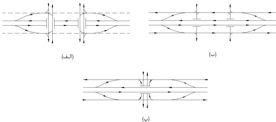
شکل ۹-۶- طرح‌های تبادلهای لوزی به منظور کاهش برخوردهای ترافیکی
