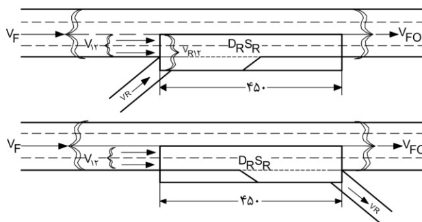
شکل ۷-۹- عوامل مختلف تأثیرگذار بر کیفیت ترافیک در ناحیه تحت تأثیر رابط
