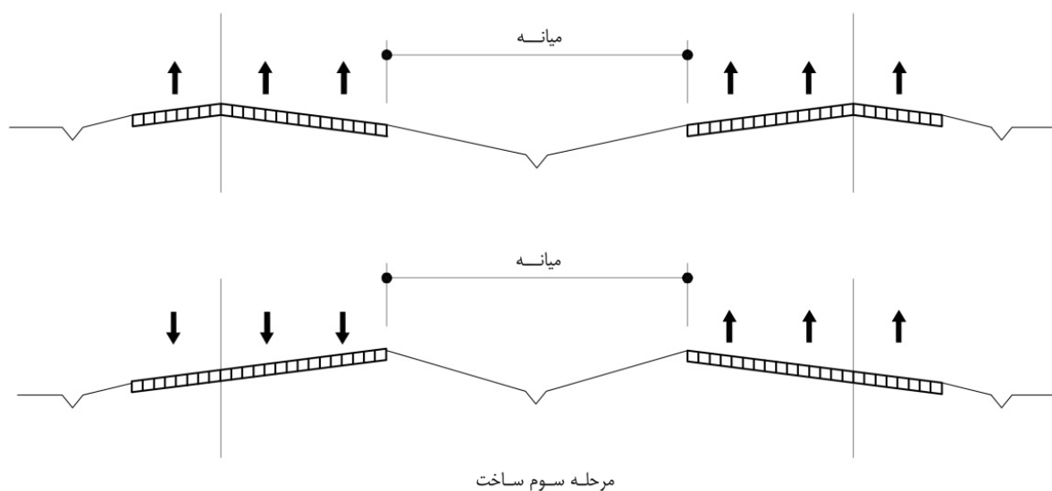
شکل ۴-۸- مرحله سوم ساخت یک راه چند خطه جداشده با میانۀ عریض
