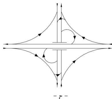
شکل ۹-۹- نمونه طرح‌های ورودی و خروجی تبادلهای نیمه‌شبدری
