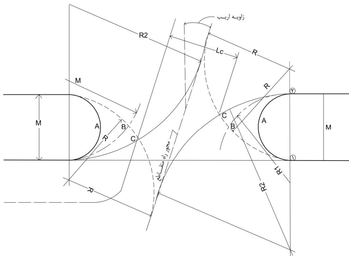
شکل ۸-۳۹- حداقل طرح بریدگی میانه و اثر اریب بودن بر آن
