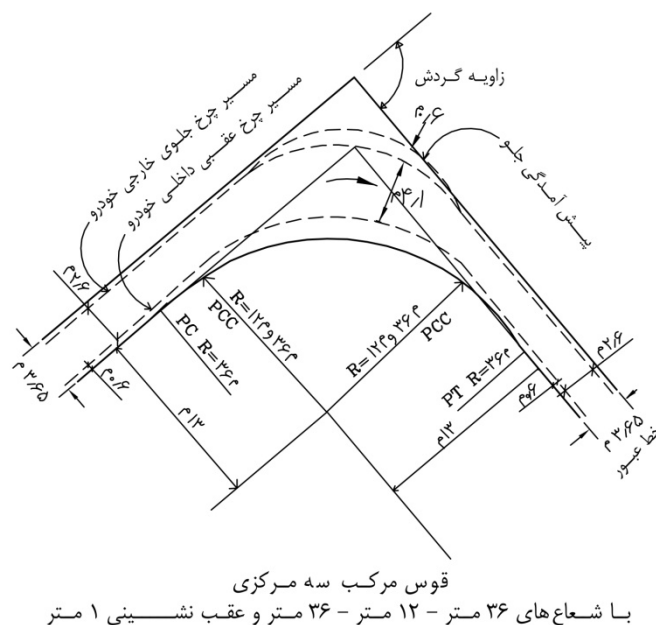
شکل ۸-۲۰- حداقل مسیر گردش برای اتوبوس نوع یک
