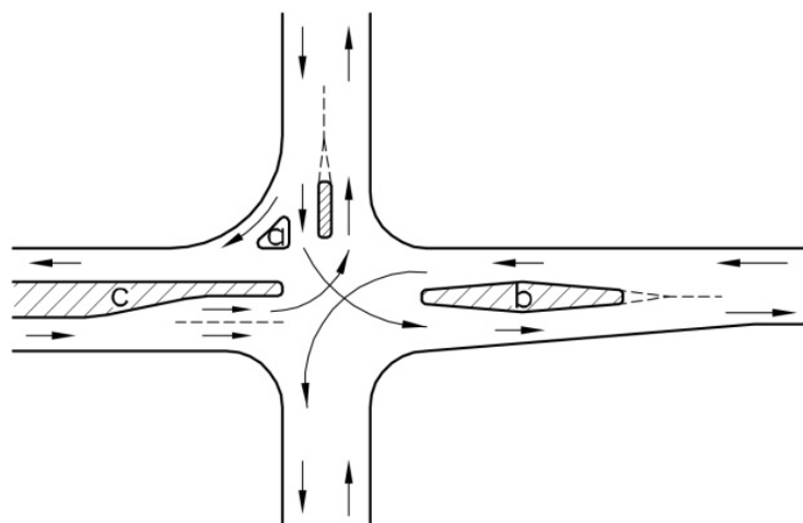
شکل ۸-۲۴- حالت متداول جزیره‌های هدایت‌کننده
