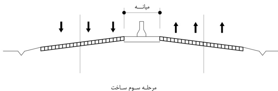
شکل ۴-۹- مرحله سوم ساخت یک راه چند خطه جداشده با میانۀ کم عرض
