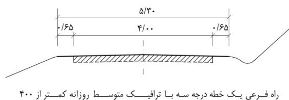
شکل ۶-۲۶- نیمرخ‌های عرضی نمونه برای راه‌های اصلی دو خطه و راه‌های فرعی
