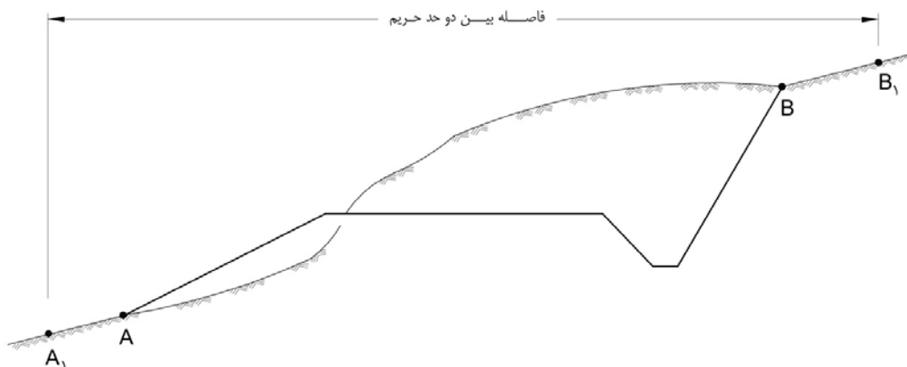
شکل ۵-۶- حریم راه
