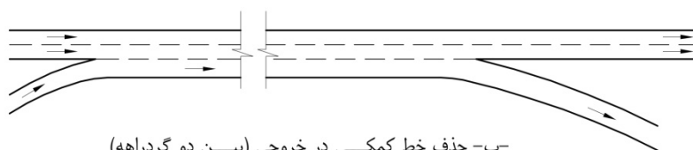
ب- حذف خط کمکی در خروجی (بین دو گردراه) و یا بین رابط‌های دو تقاطع نزدیک به هم
