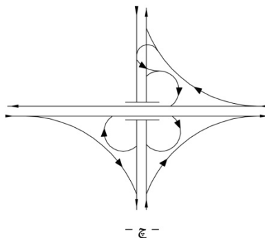
شکل ۹-۹- نمونه طرح‌های ورودی و خروجی تبادلهای نیمه‌شبدری
