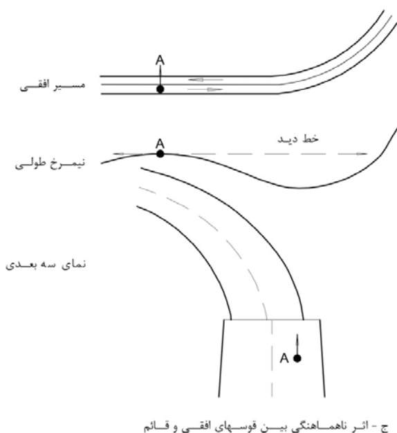
شکل ۵-۱۷- نمونه‌هایی از نحوه هماهنگی پلان و پروفیل طولی راه
