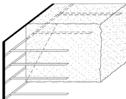
شکل ۶-۱۷- خاک مسلح
