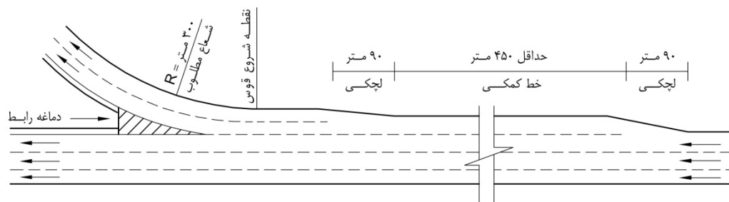
ب) طرح موازی
