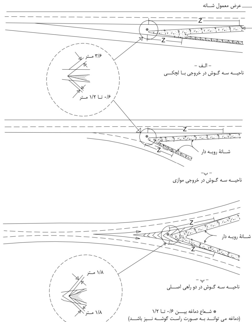
شکل ۹-۲۲- طرح‌های ناحیه سه گوش برای حالت‌های مختلف
