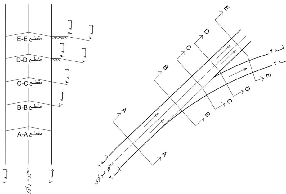
شکل ۸-۲۹- نحوه تأمین بربلندی در پایانه- جداشدگی از خط مستقیم
