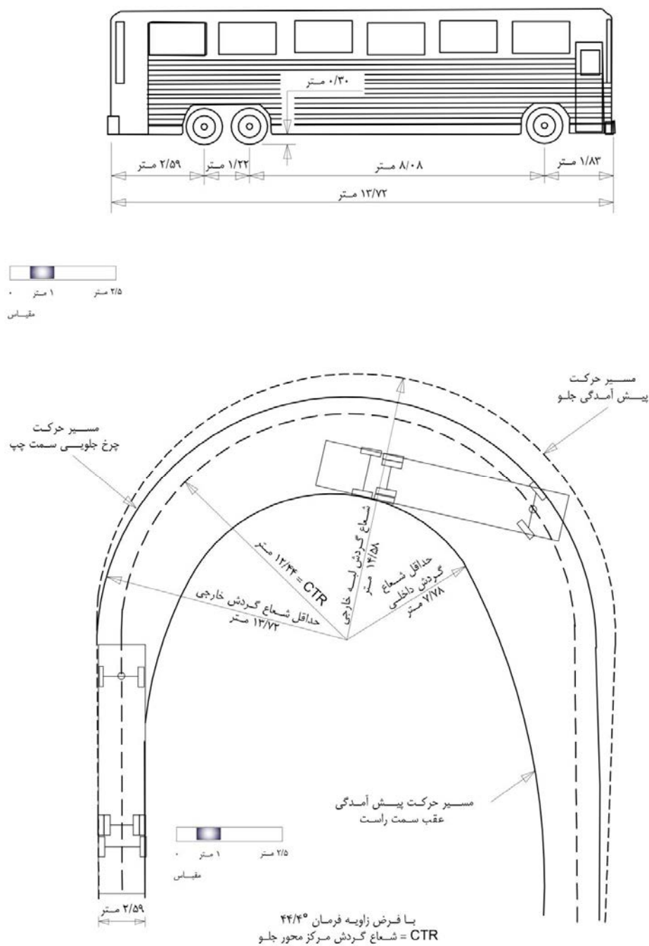
شکل ۴-۳- مشخصات مسیر گردش خودروی طرح، اتوبوس نوع دوم
