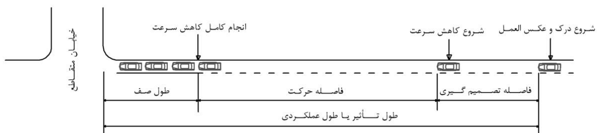
شکل ۸-۲- اجزای فضای عملکردی یک تقاطع
