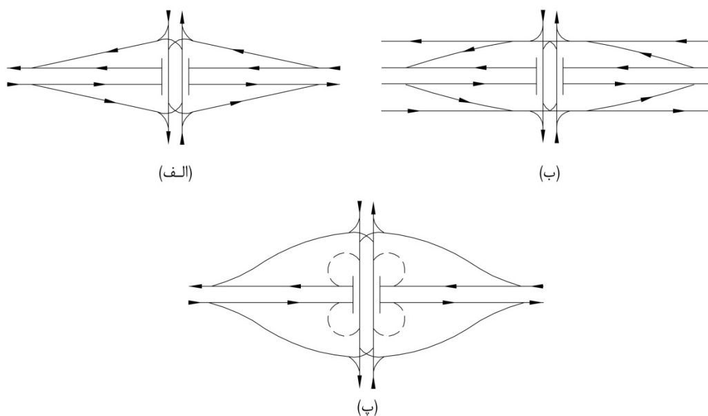
شکل ۹-۵- انواع ساده تبادلهای لوزی
