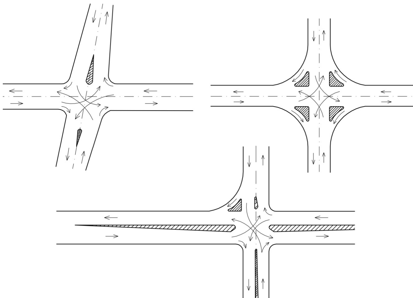
شکل ۸-۱۲- انواع طرح‌های معمول برای تقاطع‌های چهارراه
