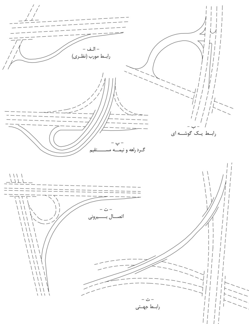
شکل ۹-۲۰- انواع مختلف رابط‌ها
