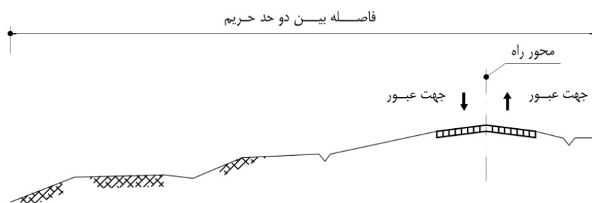
شکل ۴-۶- مرحله اول ساخت یک راه چند خطه جداشده
