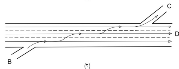
شکل ۷-۶- ناحیه تداخلی نوع ج
