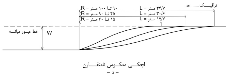
شکل ۸-۴۳- طرح لچکی برای خط کمکی
