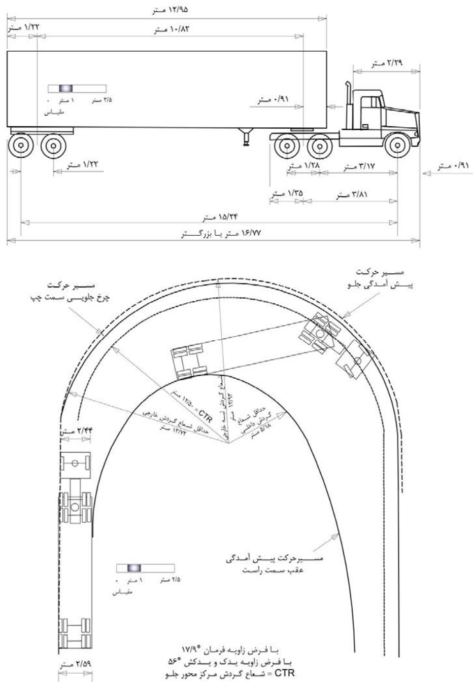
شکل ۴-۴ - مشخصات مسیر گردش خودروی طرح، کامیون نوع اول
