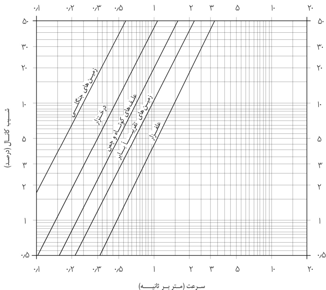
شکل ۱۰-۲- روش آپلند برای تعیین زمان حرکت آب در آبراهه کوچک تا رسیدن به کانال باز یا مجموع زمان حرکت آب به صورت ورقه‌ای و زمان حرکت آب در آبراهه کوچک تا رسیدن به کانال باز
