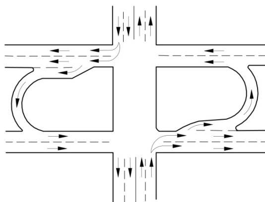
شکل ۸-۴۲- طرح مسیرهای گردش به چپ غیر مستقیم در راه‌های با میانه عریض
