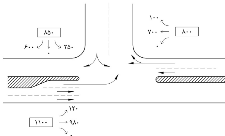
شکل ۸-۵۳- طرح شماتیک یا قیاسی اطلاعات ترافیکی تقاطع
