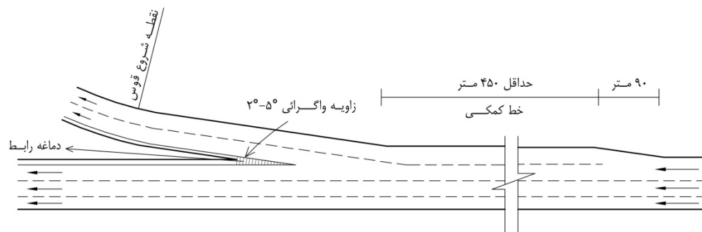
الف) طرح لچکی مستقیم
